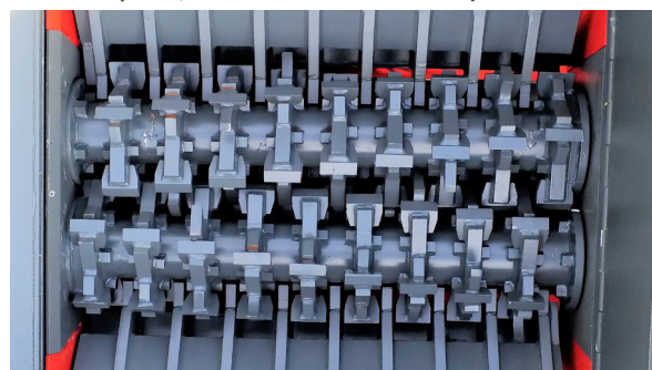
Zerkleinerungswellen: 2.000 mm
